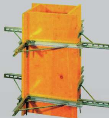
Ξυλότυποι κολώνας
